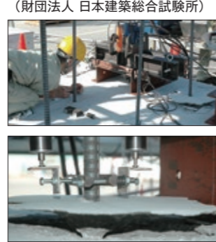
■引張試験状況 (財団法人 日本建築総合試験所)
