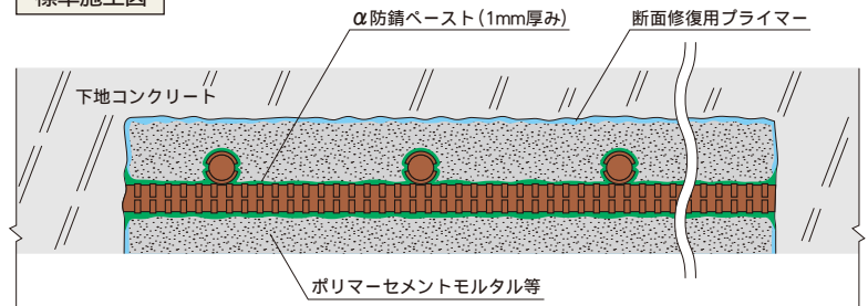
標準施工図
