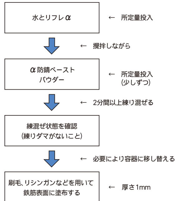
施工フロー
